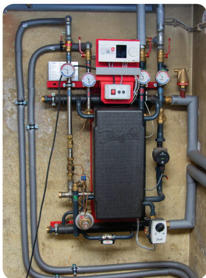
➤ Instalacja geotermalna
