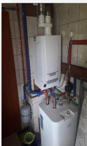
Wymiennik geotermalny
